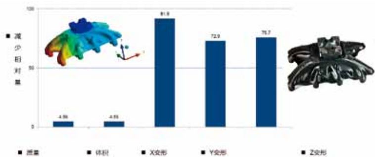
图 8 分流器封盖设计效果及实际试验情况
