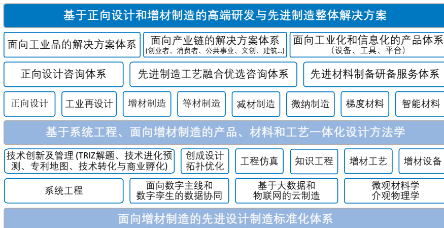
图 1 基于正向设计和增材制造的高端研发与先进制造整体解决方案技术架构
